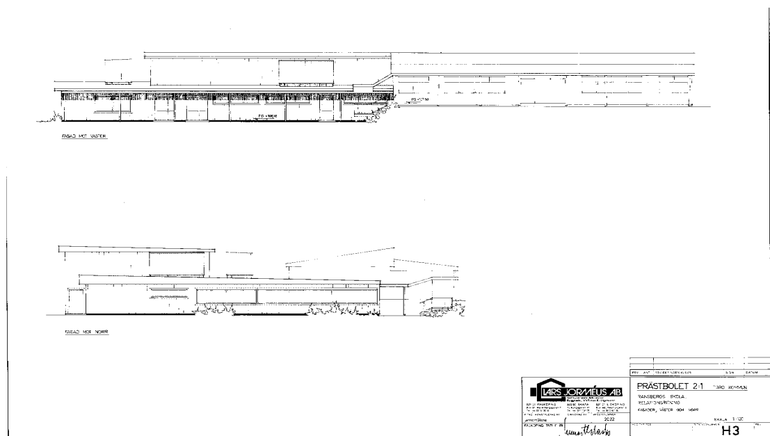
Ritning på utbyggnad från 1970-talet. Mat- och gymnastiksal. Källa: Tibro kommun stadsarkiv, stadsbyggnadsenheten.
